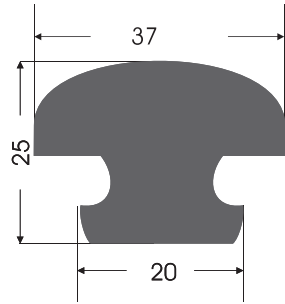
TL - 0002 İÇ TAMBUR LASTİĞİ INSIDE MAINWINCH RUBBER
