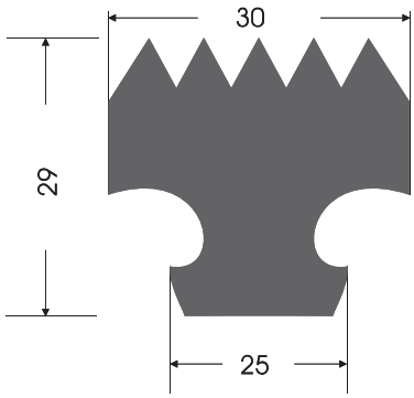
TL - 0001 İÇ TAMBUR LASTİĞİ INSIDE MAINWINCH RUBBER
