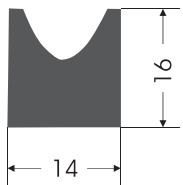
KC - 0017 KAPAK CONTASI COVER GASKET
