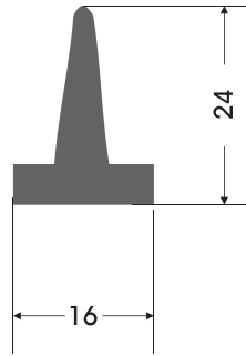
SL - 0006 SIYIRICI LASTIĞI STRIPPING OFF RUBBER
