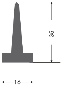
SL - 0005 SIYIRICI LASTIĞI STRIPPING OFF RUBBER
