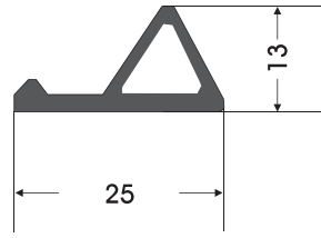
RC - 0005 RAMÖZ CONTASI STENTER GASKET
