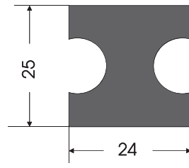
TL - 0003 İÇ TAMBUR LASTİĞİ INSIDE MAINWINCH RUBBER
