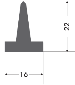
SL - 0003 SIYIRICI LASTIĞI STRIPPING OFF RUBBER
