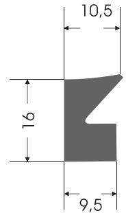
KC - 0016 KAPAK CONTASI COVER GASKET
