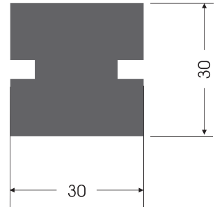
TL - 0016 İÇ TAMBUR LASTİĞİ INSIDE MAINWINCH RUBBER
