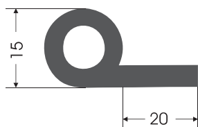
PP - 0010 P PROFIL P PROFIL
