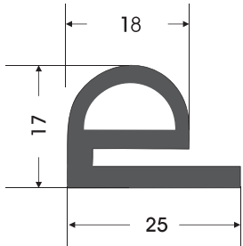
RC - 0008 RAMÖZ CONTASI STENTER GASKET
