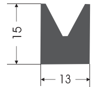
KC - 0016 KAPAK CONTASI COVER GASKET
