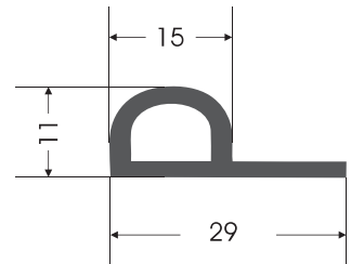
PP - 0008 P PROFIL P PROFIL
