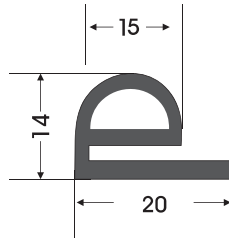
RC - 0009 RAMÖZ CONTASI STENTER GASKET
