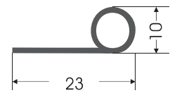
PP - 0012 P PROFIL P PROFIL
