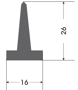
SL - 0004 SIYIRICI LASTIĞI STRIPPING OFF RUBBER
