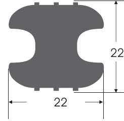
TL - 0003 İÇ TAMBUR LASTİĞİ INSIDE MAINWINCH RUBBER
