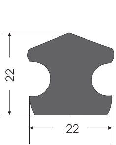
TL - 0013 İÇ TAMBUR LASTİĞİ INSIDE MAINWINCH RUBBER
