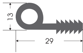
PP - 0002 P PROFIL P PROFIL
