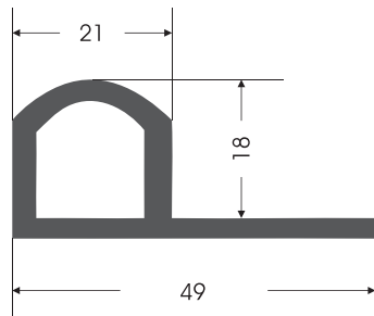
PP - 0006 P PROFIL P PROFIL
