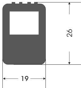
CL - 0002 KON, YIKAMA CAM LAS. WASHING GLASS RUBBER
