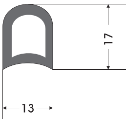
RC - 0001 RAMÖZ CONTASI STENTER GASKET
