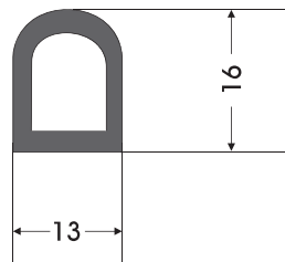
RC - 0002 RAMÖZ CONTASI STENTER GASKET
