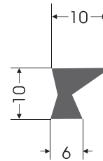
KC - 0015 KAPAK CONTASI COVER GASKET
