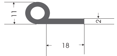
PP - 0004 P PROFIL P PROFIL
