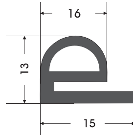
RC - 0010 RAMÖZ CONTASI STENTER GASKET
