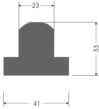
TL - 0015 İÇ TAMBUR LASTİĞİ INSIDE MAINWINCH RUBBER
