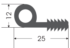
PP - 0001 P PROFIL P PROFIL
