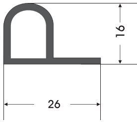
RC - 0004 RAMÖZ CONTASI STENTER GASKET
