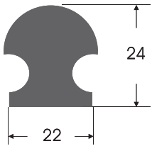
TL - 0009 İÇ TAMBUR LASTİĞİ INSIDE MAINWINCH RUBBER
