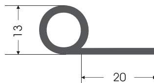
PP - 0011 P PROFIL P PROFIL
