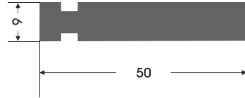
SL - 0002 SIYIRICI LASTIĞI STRIPPING OFF RUBBER
