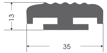
KL - 0002 KUMAŞ KONTROL LASTIĞI STUFF CONTROL RUBBER
