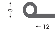
PP - 0003 P PROFIL P PROFIL
