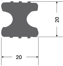
TL - 0005 İÇ TAMBUR LASTİĞİ INSIDE MAINWINCH RUBBER
