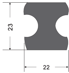
TL - 0006 İÇ TAMBUR LASTİĞİ INSIDE MAINWINCH RUBBER
