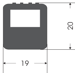
CL - 0003 KON, YIKAMA CAM LAS. WASHING GLASS RUBBER
