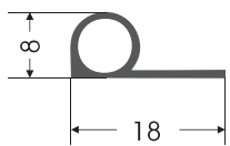
PP - 0009 P PROFIL P PROFIL
