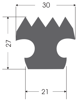
TL - 0014 İÇ TAMBUR LASTİĞİ INSIDE MAINWINCH RUBBER
