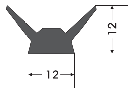
RC - 0003 RAMÖZ CONTASI STENTER GASKET
