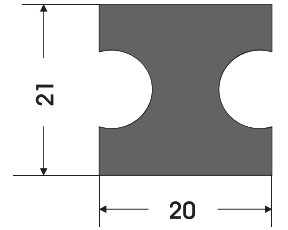
TL - 0004 İÇ TAMBUR LASTİĞİ INSIDE MAINWINCH RUBBER
